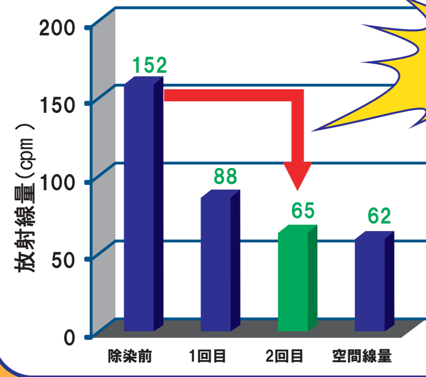
ALOKA製TGS-146Bを用いて表面汚染を測定
